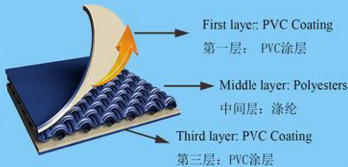
PVC Fabric Coated Tarp Component PVC 夹网布结构图
